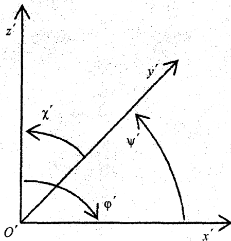
Рисунок Б.1 – Степени свободы фундамента
